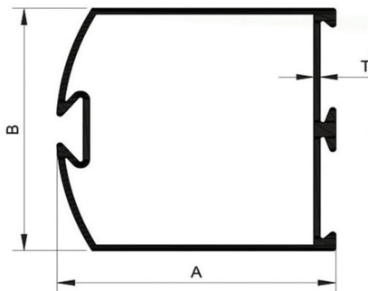
47 X 44 DOOR TOP
