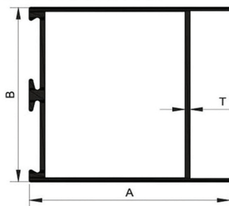
47 X 44 DOOR TOP
